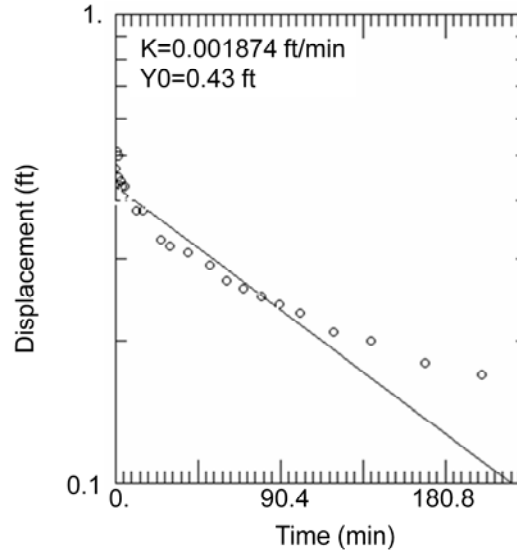
LNAPL Baildown Test Example; MW-6
