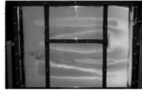
L. Donor., T. Sale, CSU
